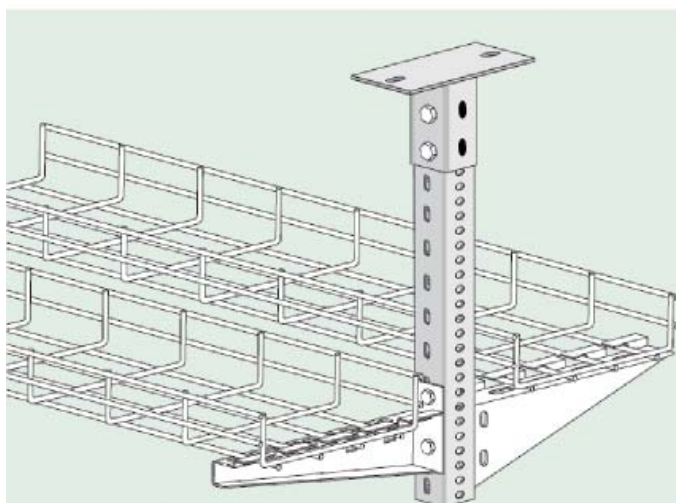
Ejemplo de montaje / Assembly sample
